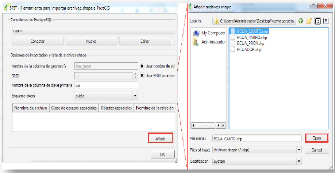
Figura 15: Añadir archivos shape.
